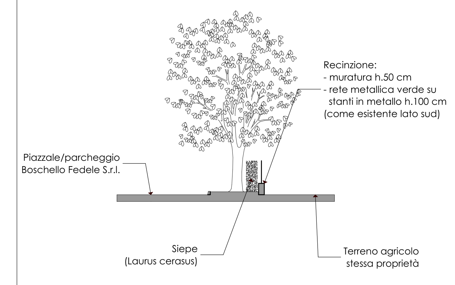
RECINZIONE TIPO "B" (lato nord e sud)
