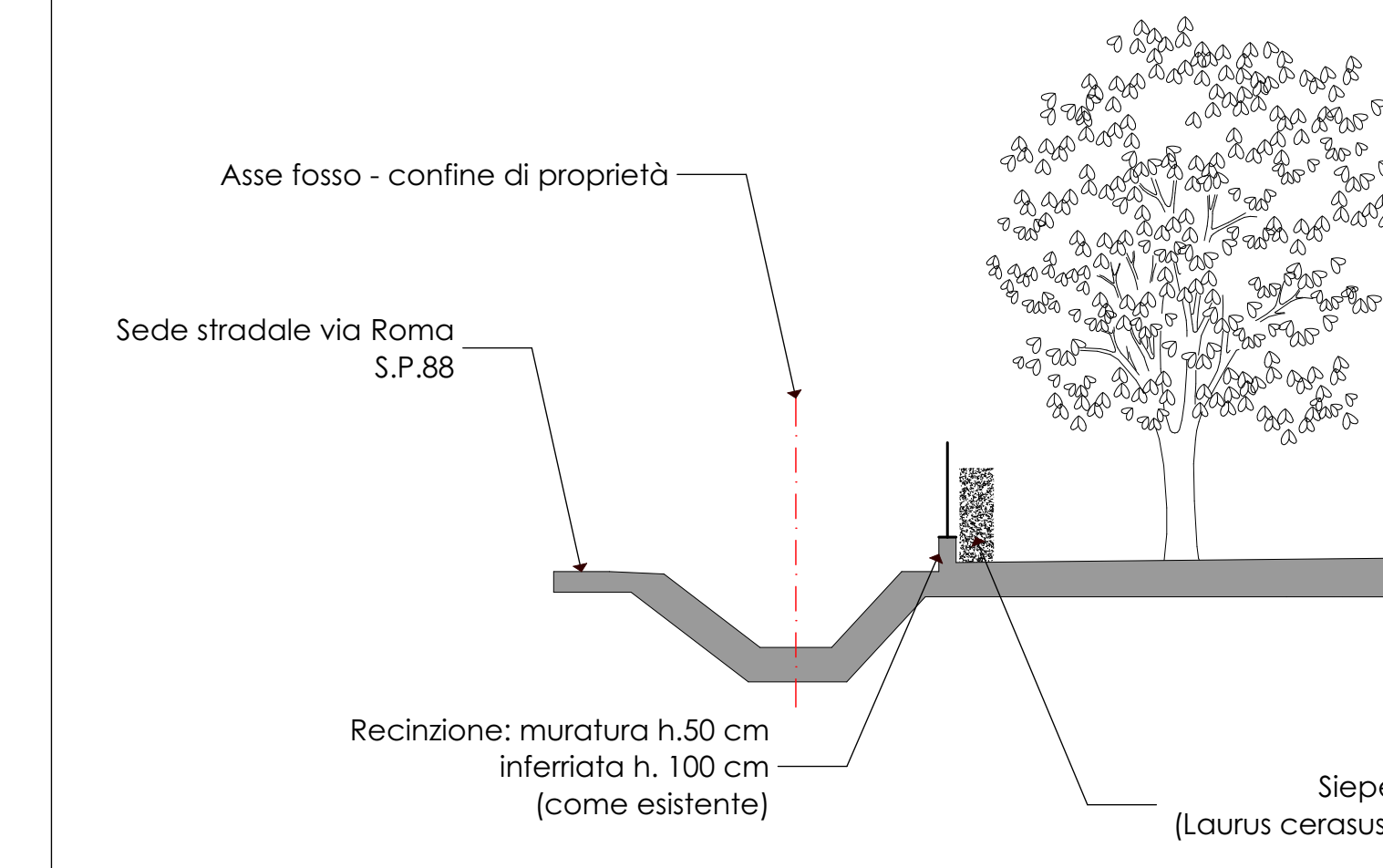
RECINZIONE TIPO "A" (lato ovest)
