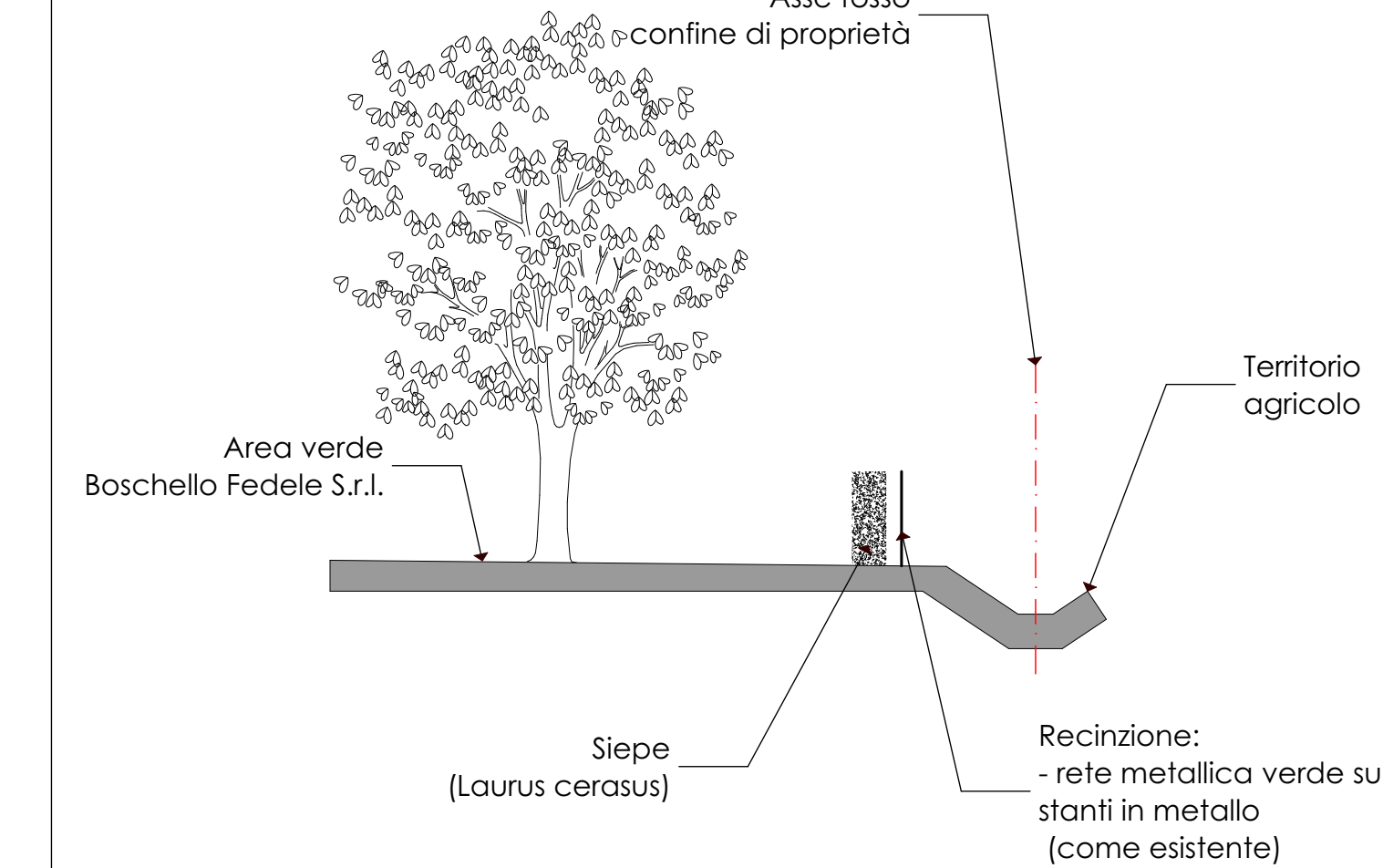
RECINZIONE TIPO "C" (lato est)
