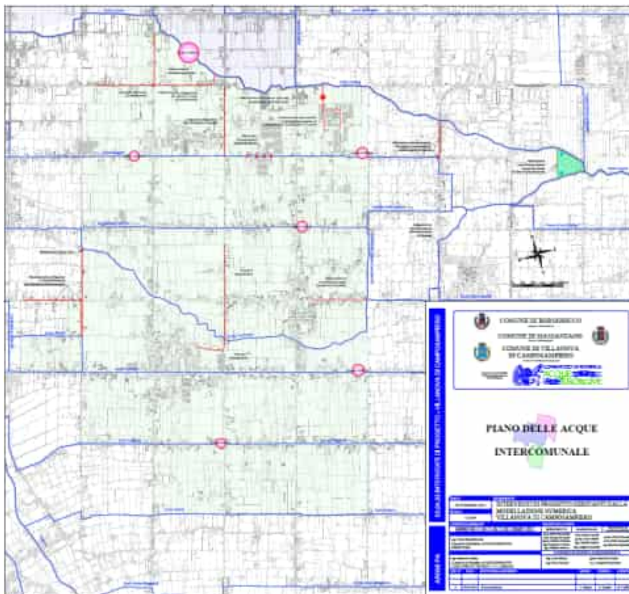
Figura 4.8: Carta degli interventi di progetto del Piano delle Acque per Villanova di Camposampiero.
