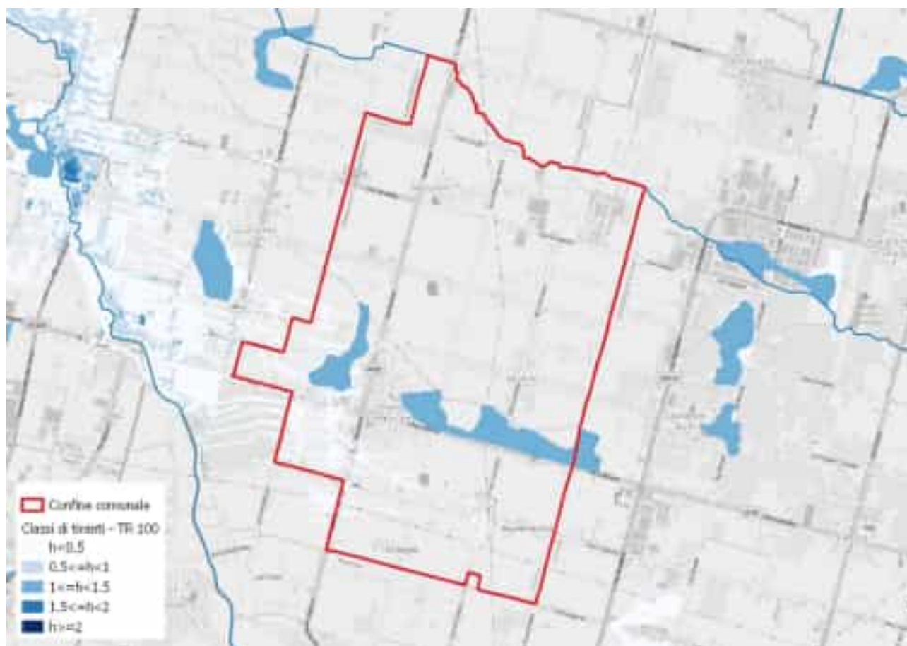
Figura 4.2: PGRA 2021-2027: aree allagabili e altezze idriche nello scenario di media probabilità (Tr=100 anni). Elaborazione GIS su dati Autorità di bacino Alpi orientali.
